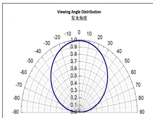
Viewing Angle Distribution 发光角度
